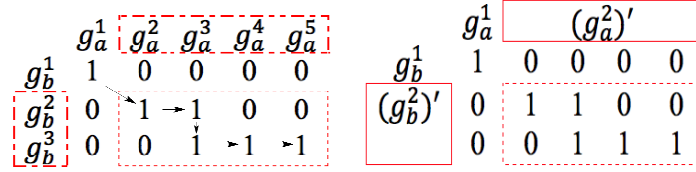
Figure 8. Illustration du processus de fusion de blocs reposant sur la distance DTW (les flèches indiquent le chemin optimal suivi pour l'appariement).
