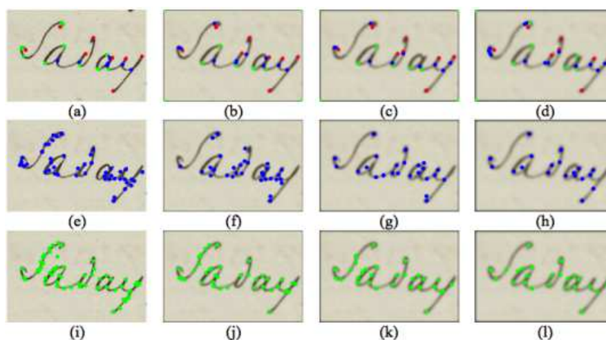
Figure 3: Trois approches de détection de points saillants (en ligne) et visualisation des résultats en fonction d'une dégradation par flou gaussien croissant. Détecteur de points de structure (ligne 1), détecteur de point DoG (ligne 2) et détecteur de points par matrice Hessienne (ligne 3)
