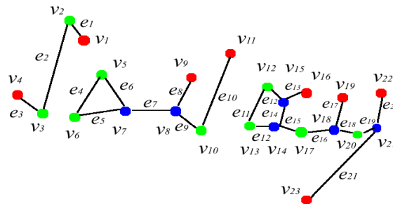
Figure 5. Représentation en une séquence de trois graphes du mot "Savay".
