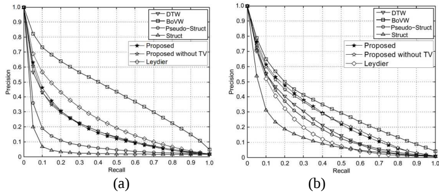
Figure 10. Courbes de précision-rappel pour 7 méthodes de word-spotting portant sur (a) la base George Washington GW et (b) le registre de mariages de la cathédrale de Barcelone 5CofM.
