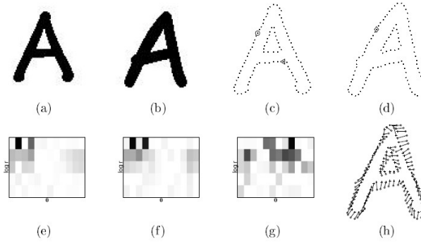
Figure 4. Illustration du descripteur de Contexte de Formes (SC) et principe de l'appariement. (a) et (b) images originales. (c) et (d) Points de contours. (e), (f) et (g) Histogrammes SC estimés à partir des trois points notés \phi , \Delta et \circ .
