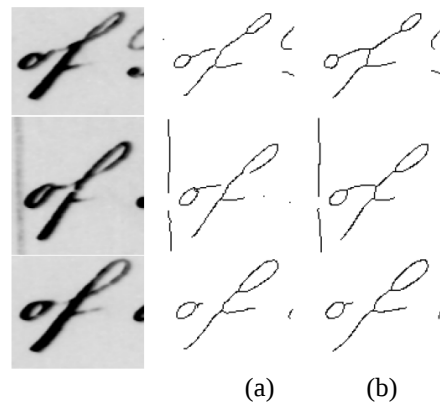
Figure 1.a. Exemples de squelettes extraits par la méthode de Zhang (Zhang et Suen, 1984) pour 3 instances d'un mot extrait de la collection George Washington, 1.b. Leur apparence après l'application du vote tensoriel sur le squelette initial.
