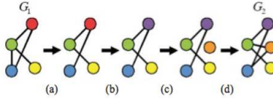
Figure 6: Exemple de chemin d'édition modélisant la transformation du graphe G_1 en graphe G_2 : (a) suppression d'arête (b) substitution de sommet (c) insertion de nœud (d) insertion d'arête.
